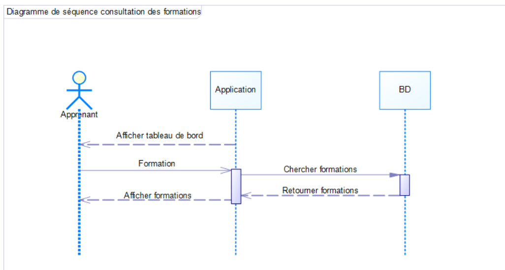
Figure 21 : Diagramme de séquence « Consultation des formations disponibles »
