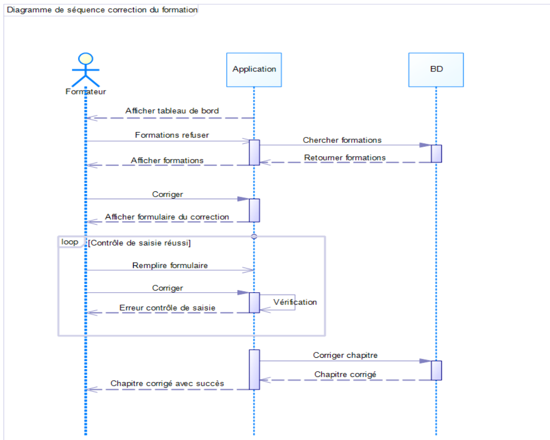
Figure 16 : Diagramme de séquence « Correction de la formation »
