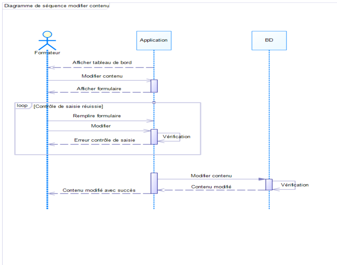
Figure 7 : Diagramme de séquence « Modification de contenu pédagogique »
