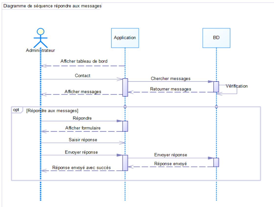
Figure 37 : Diagramme de séquence « Gestion des messages »
