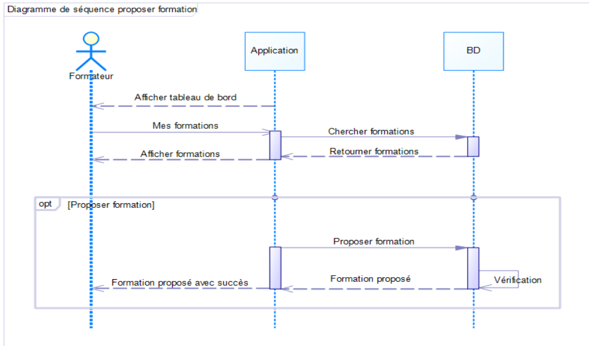
Figure 9 : Diagramme de séquence « Proposition de la formation à l'expert »
